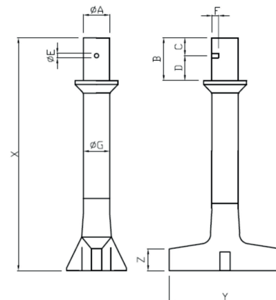
T-BAR STIRRERS
